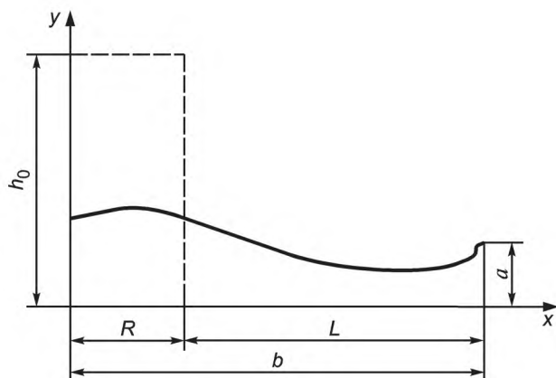
Рисунок К.2 — Типичная картина движения жидкости в обваловании при мгновенном разрушении резервуара - - - - - уровень начального столба жидкости; ———— уровень жидкости в промежуточный момент времени (результаты расчета)
