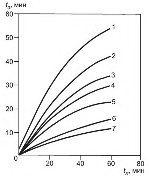
Рисунок Р.6 — Зависимость эквивалентной продолжительности пожара t_3 от продолжительности пожара t_n для вертикальных незащищенных металлических конструкций
